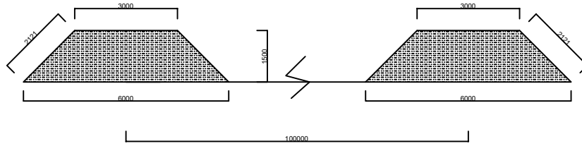
蓄水池剖面图
