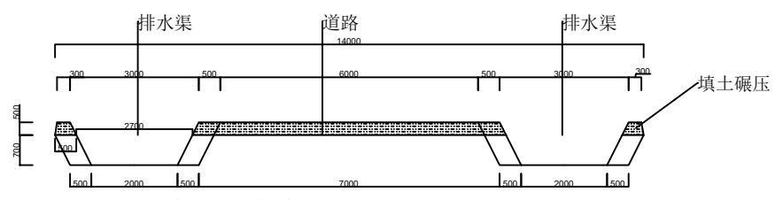
排水渠及道路剖面图
