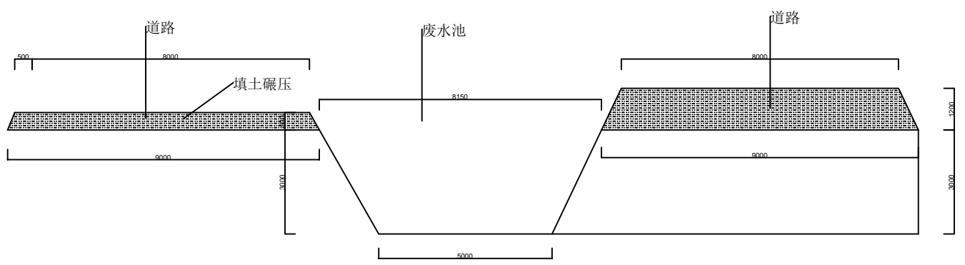
排水渠及废水池剖面图
