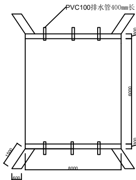
平面图
