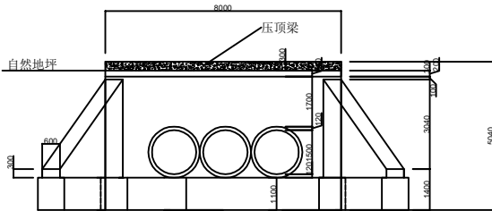
立面图
