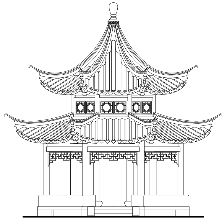
十六柱八角重檐亭立面图1:50
