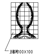
宝顶大样1:25
