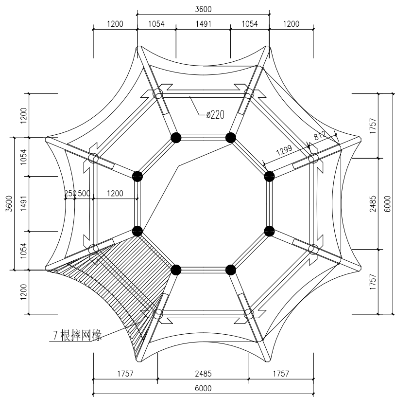
下沿屋架平面图1:50
