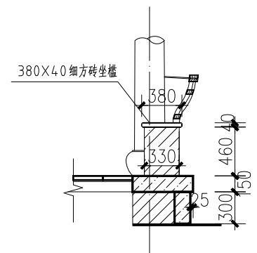
坐槛大样1:25
