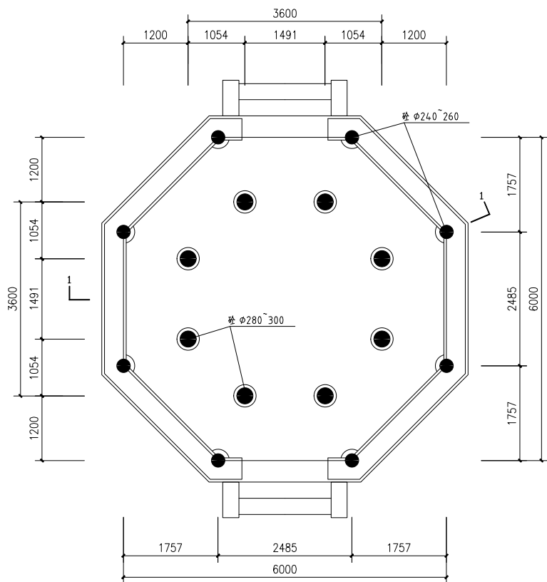
十六柱八角重檐亭平面图1:50
