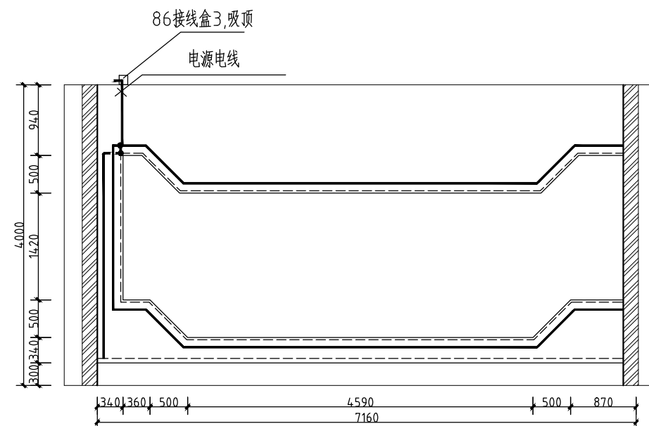
② 二层铁人精神展厅立面照明图 1:50
