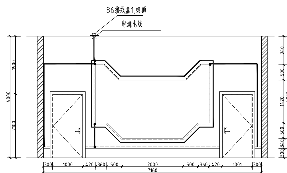
④ 二层铁人精神展厅立面照明图 1:50
