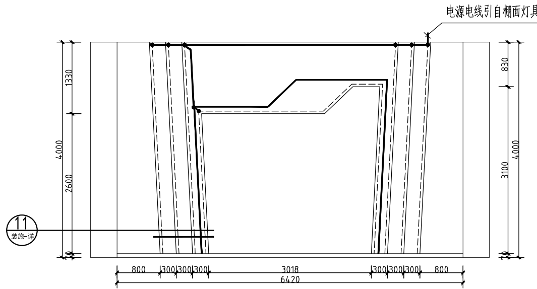
⑪ 二层典型模范榜样区展开立面照明图 1:50
