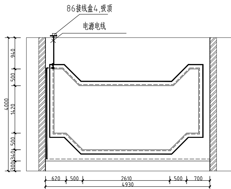
① 二层铁人精神展厅立面照明图 1:50
