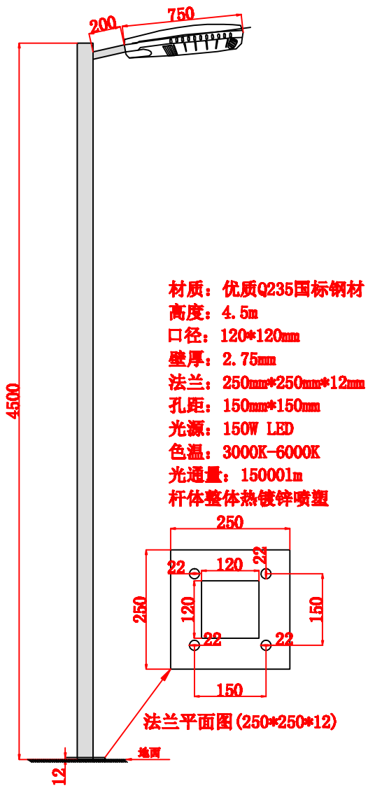
4.5米路灯立面图
