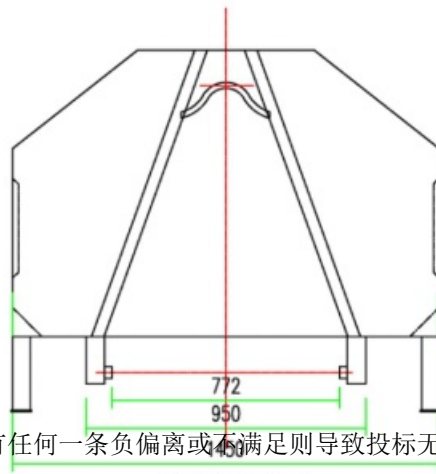
钩臂箱配套尺寸
