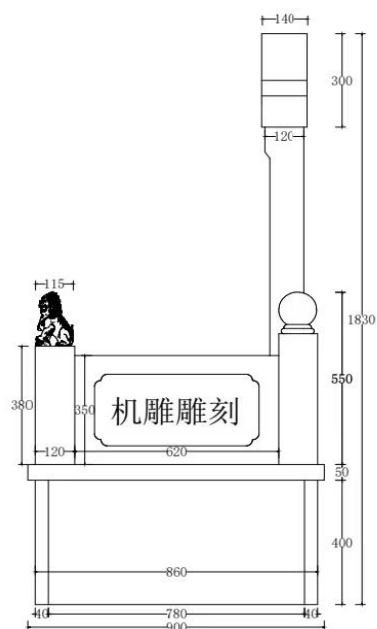
侧面图
