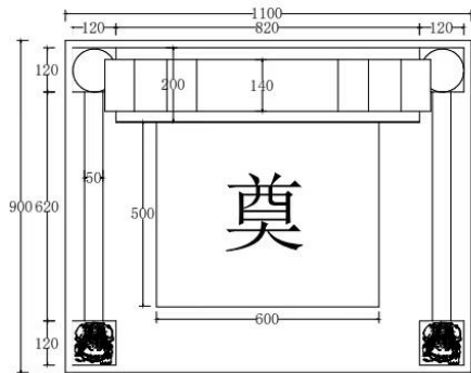
平面图
