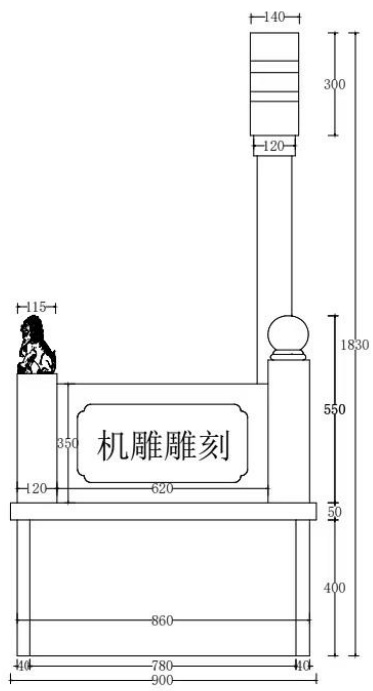
侧面图
