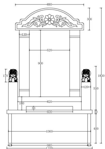
正面图
