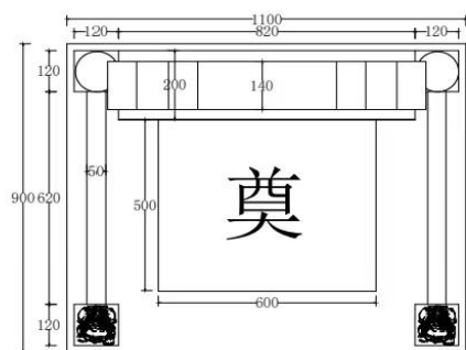
平面图
