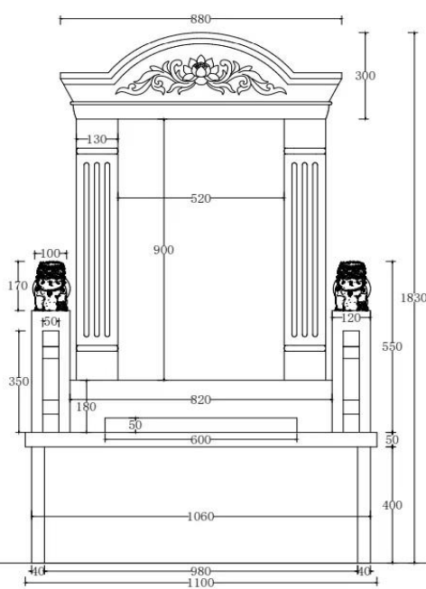
正面图
