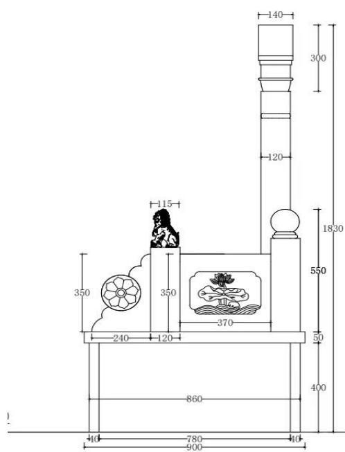
侧面图
