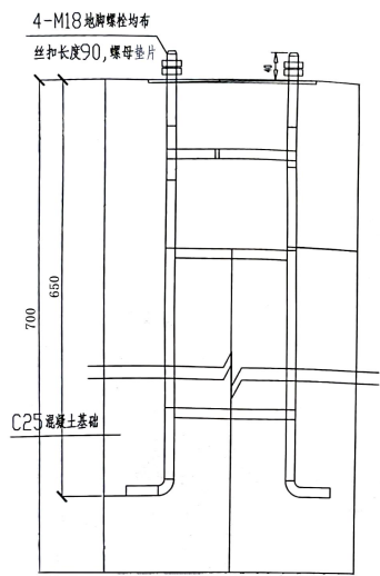
路灯基础做法详图
