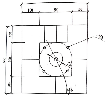
路灯基础平面图
