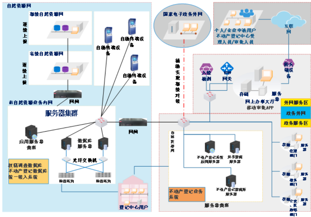
图1机房环境部署图
