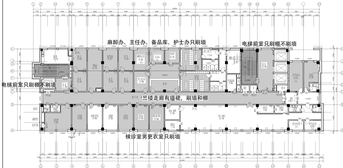
三层平面图 1:100
