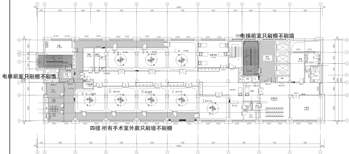
四层平面图 1:100 建筑面积: 1256.54m 2
