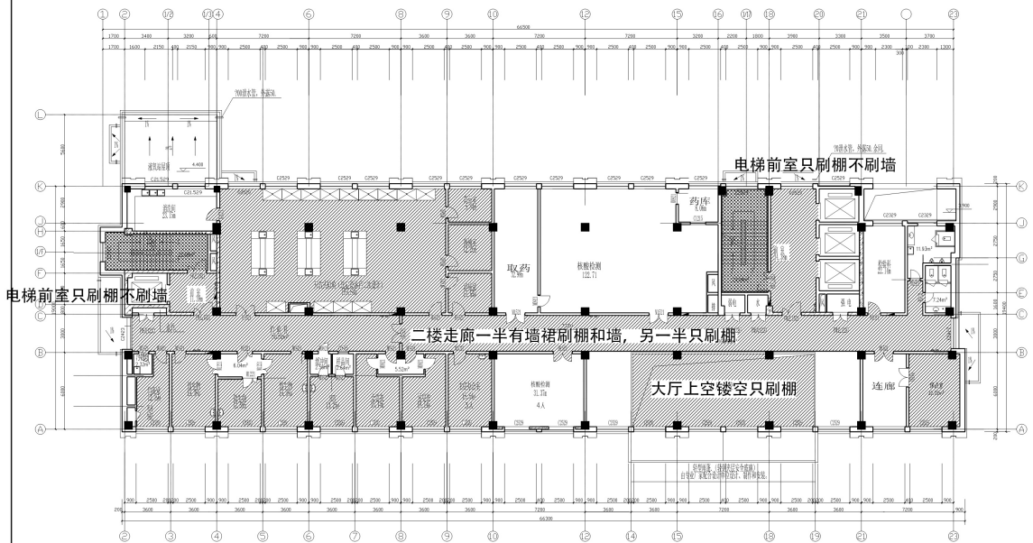
二层平面图 1:100 建筑面积: 1256.54m 2
