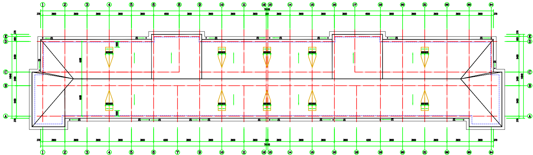
28.28.48.78 屋面平面图 1:100
